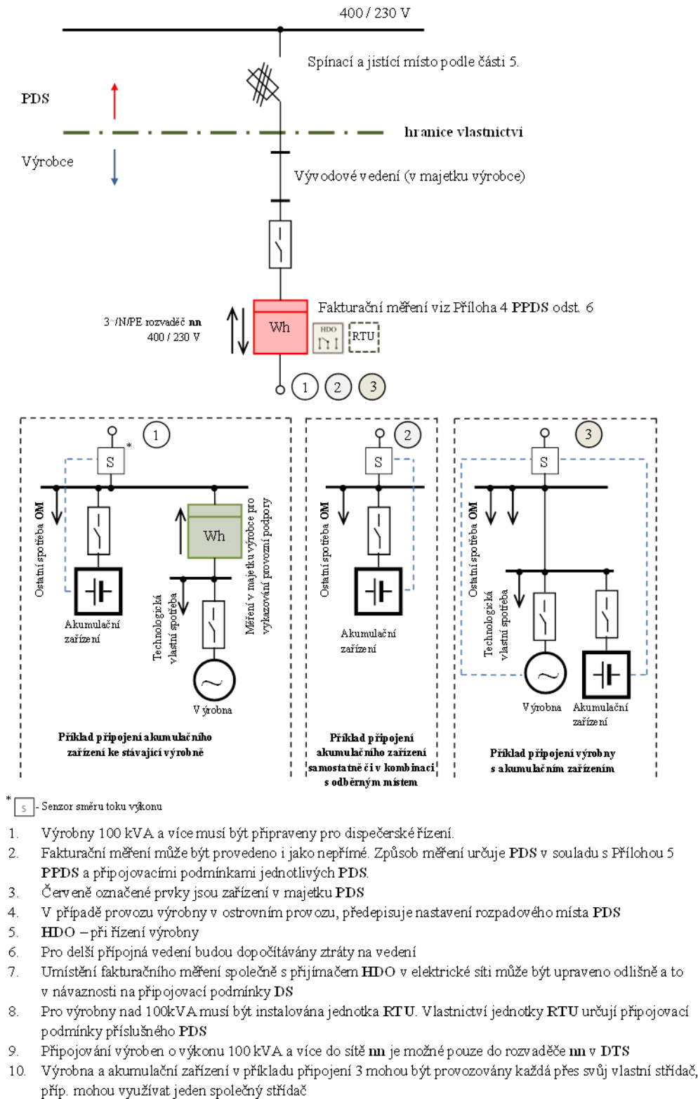
Obr. 22 Připojení výroby s akumulčním zařízením nn
